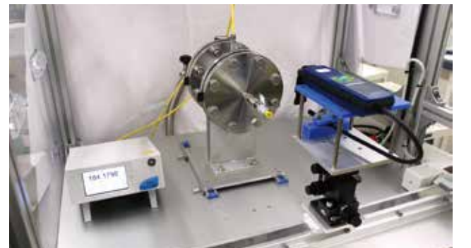
試験装置
