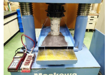
静弾性係数試験
