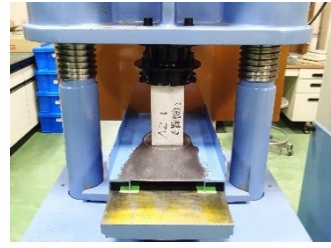
ボス供試体圧縮試験
