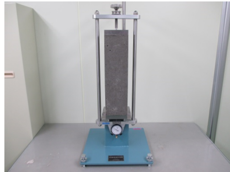
写真2 測長状況
