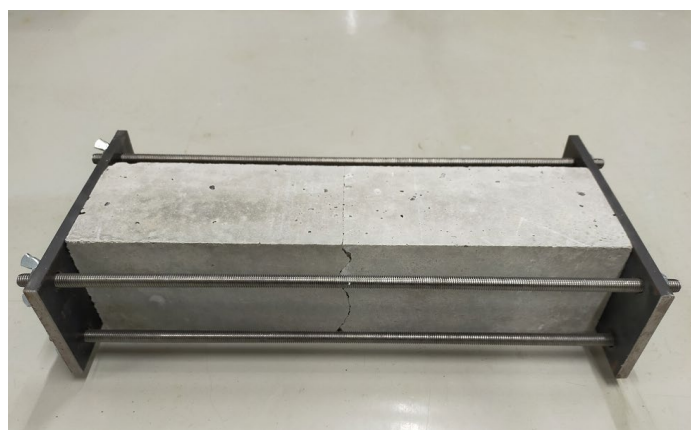
0.2 mm固定状況
