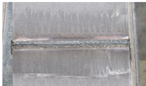
突合せ溶接供試体
