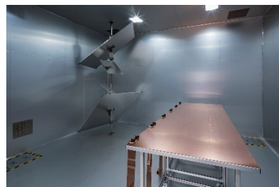
高周波までの安定した試験が行えるリバレーションチャンバー
